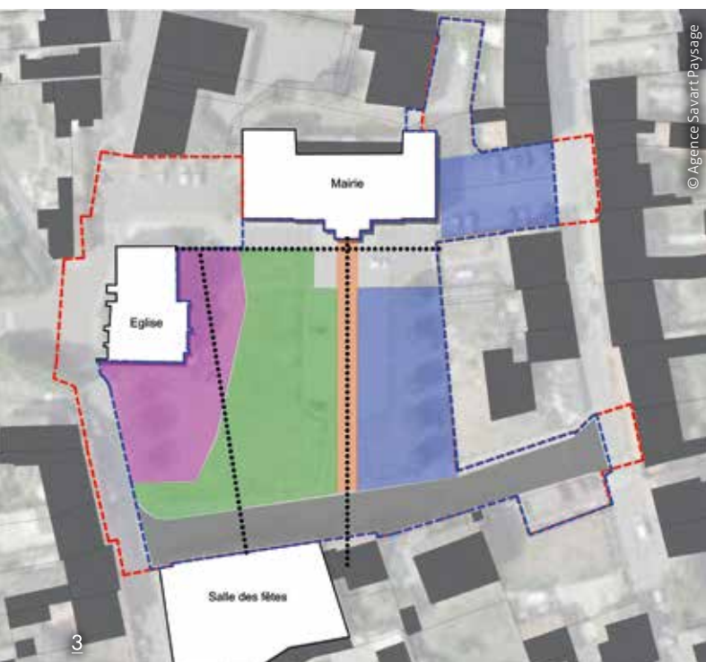
3/ La conception s'appuie sur les axes de composition immuables du site (en noir) et s'organise autour de trois entités successives : les parkings (en bleu), le jardin (en vert) et la figuration de l'ancien cimetière communal (en rose). 4/ Le jardin est conçu comme un tissu végétal, composé de trames de rosiers paysagers, de graminées, de vivaces, de banquettes régulières et de surfaces enherbées qui s'entrelacent, en référence à l'histoire des anciennes filatures présentes sur le territoire.
